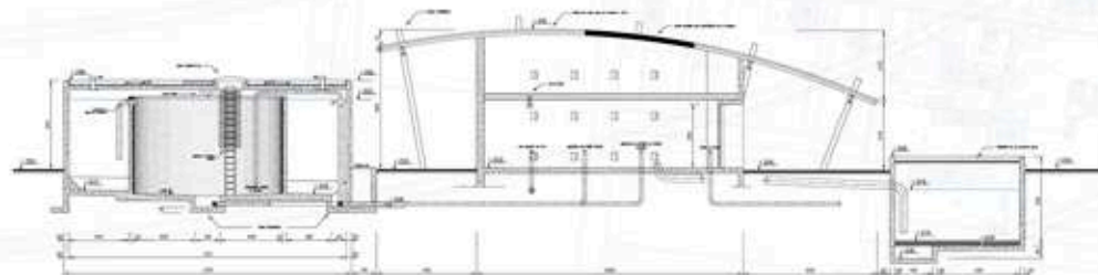
COUPE A-A
